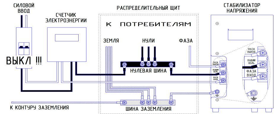
Рисунок 1. Рекомендуемая схема подключения стабилизатора к сети.
